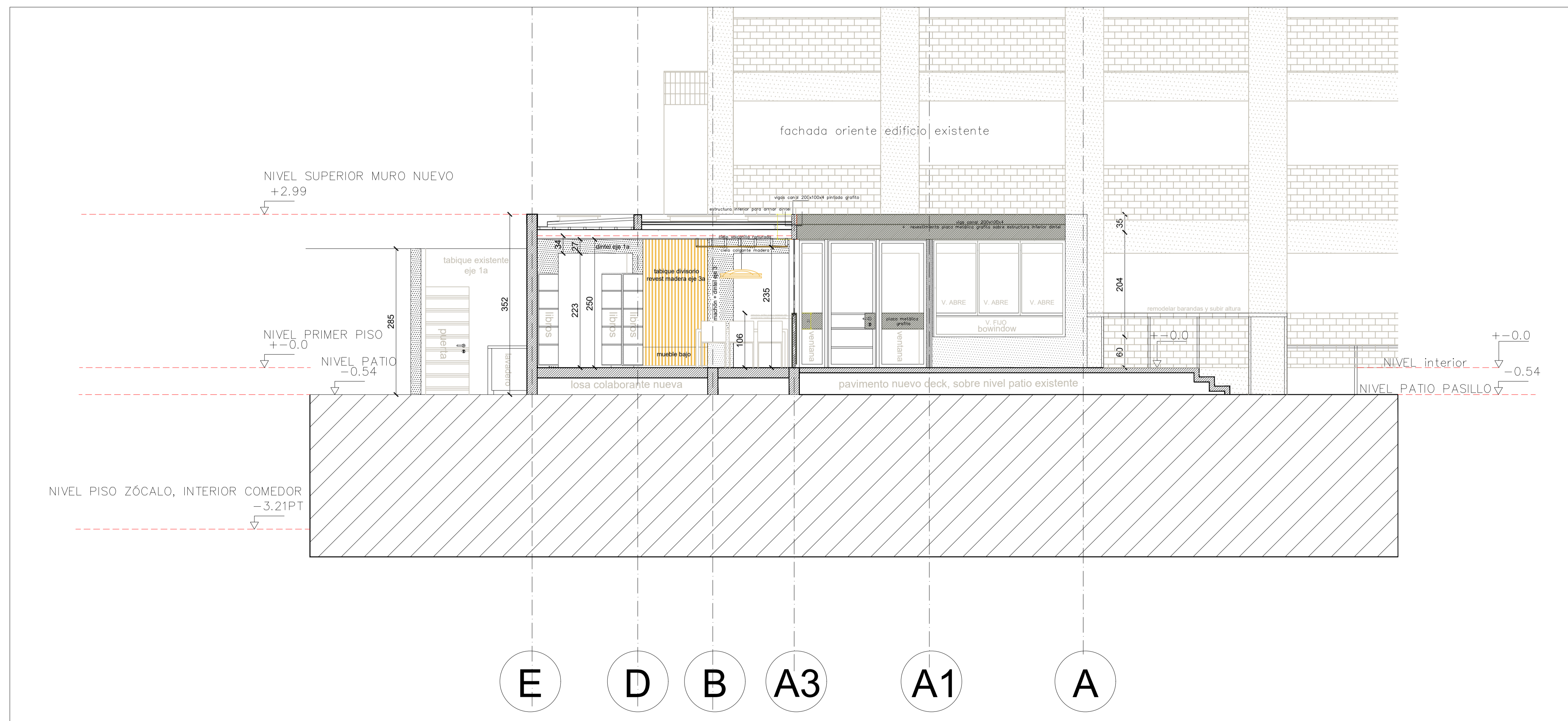
BIBLOTECA FACHADA ORIENTE - CORTE D-D" / ESCALA 1:50
