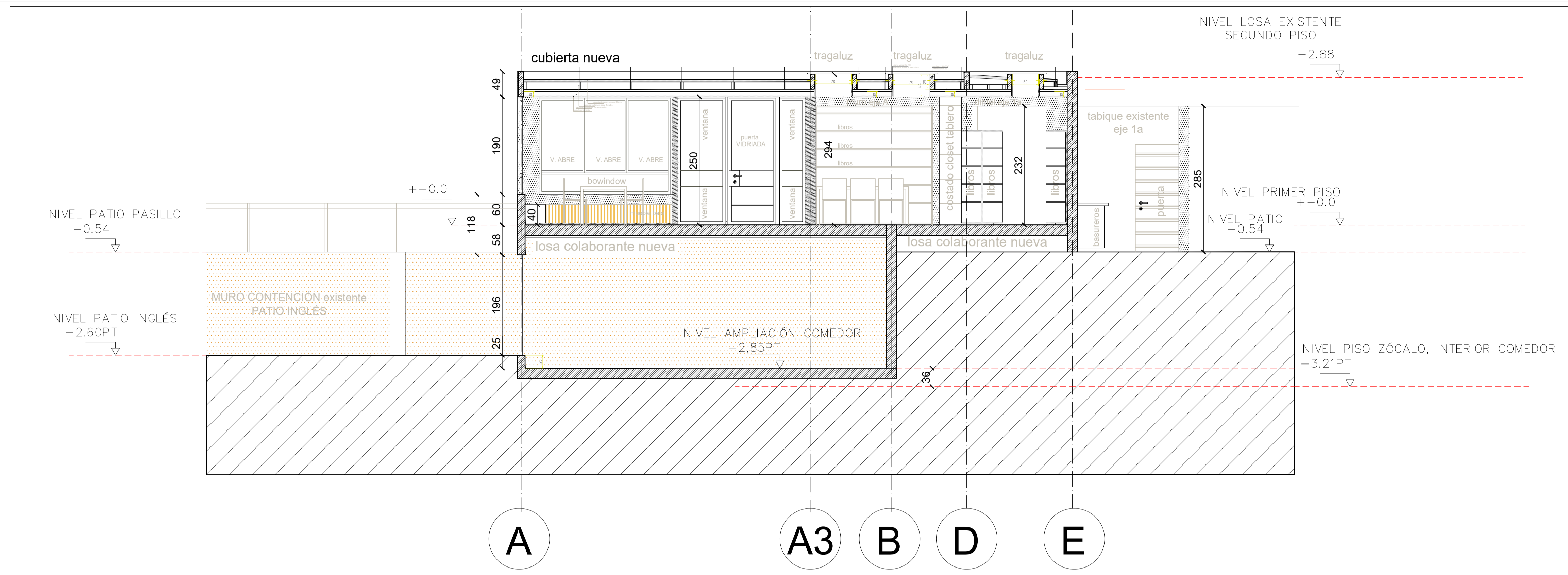
BIBLOTECA CORTE C-C" / ESCALA 1:50
