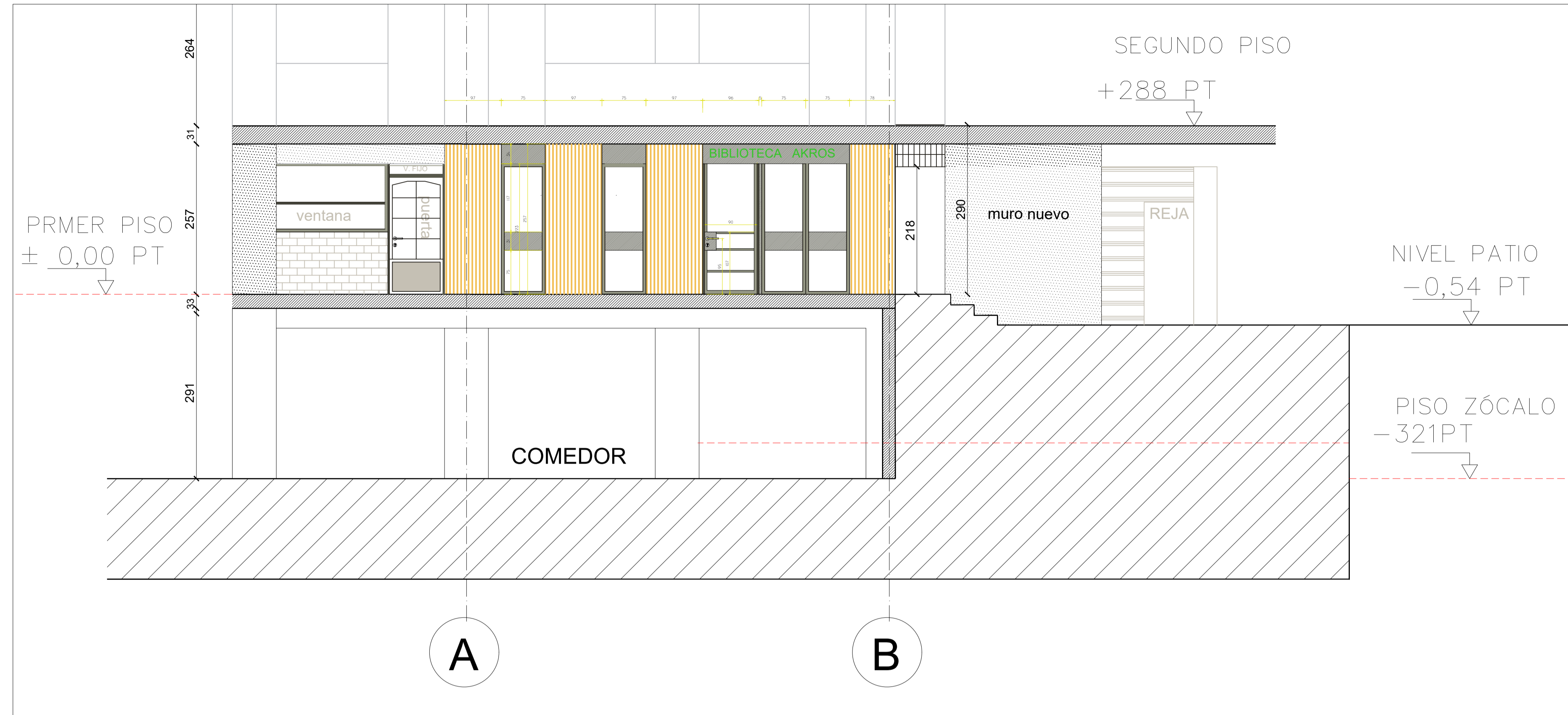
BIBLIOTECA/ FACHADA PONIENTE HACIA PATIO PRINCIPAL / ESCALA 1:50
