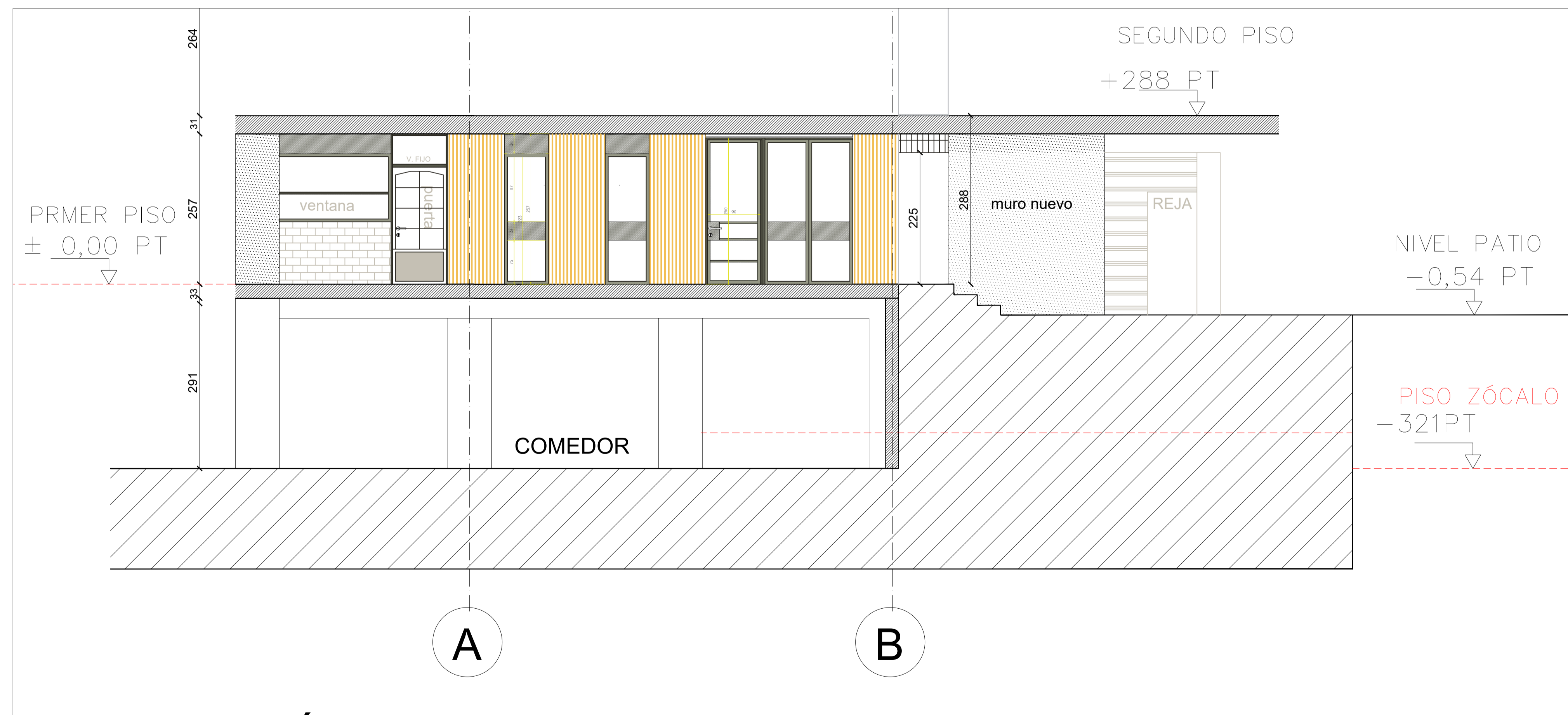
BIBLIOTECA/ FACHADA PONIENTE INTERIOR PASILLO / ESCALA 1:50
